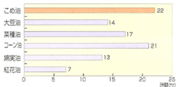
植物性油脂の酸化安定性(AOM試験)
